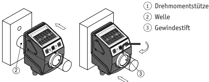
Abb. 2: Montage
