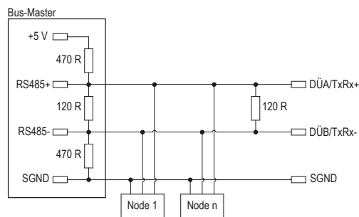
Abb. 3: Terminierung und Pegelfestlegung RS485
