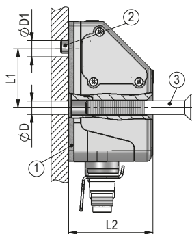
Abb. 1: Einbaumaße
