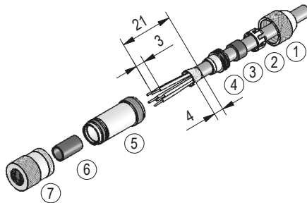
Abb. 6: Gegenstecker M8 gerade
