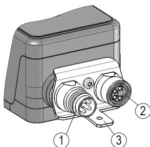
Abb. 4: Anschlussbelegung
