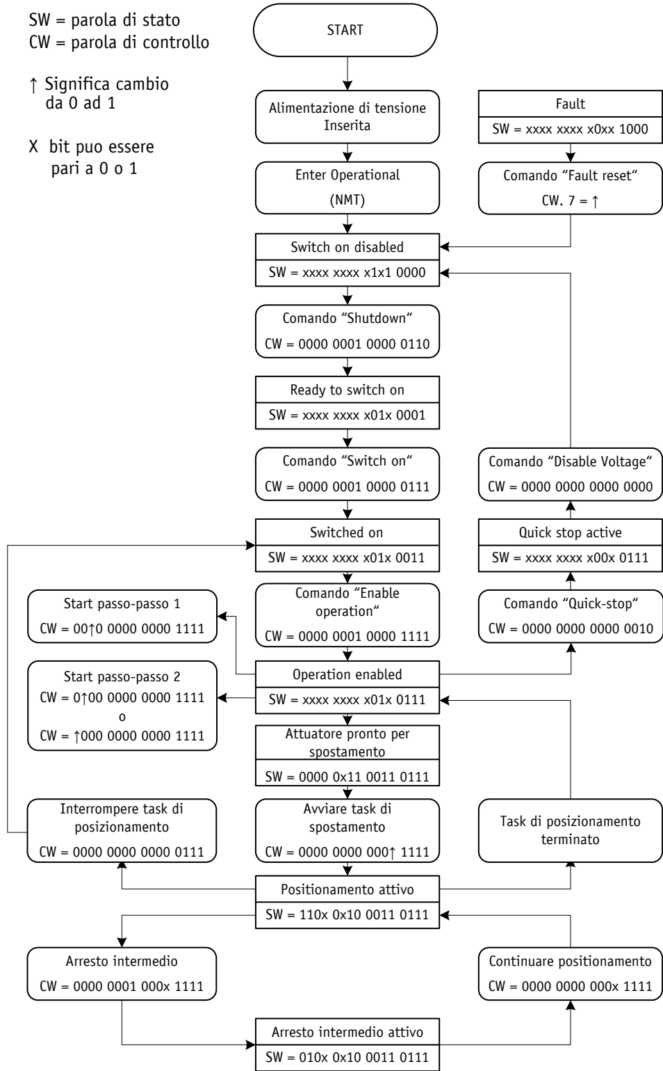
Fig. 30: flow chart modo operativo Profile Position Mode (modo Posizionamento)
