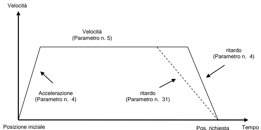
Fig. 2: rampa con modo Posizionamento (diretta)
